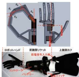
図1 日常生活に必要な基本3種の把持姿勢がとれる実用型筋電義手
