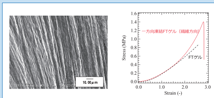
図1 一方向凍結法による凍結解凍ゲルのフィブリルの様子(左)と引張強度(右)
